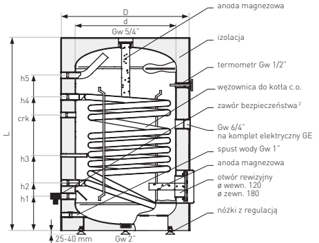
Wymiennik Etna 200
