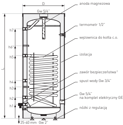
Wymiennik Etna 100-140
